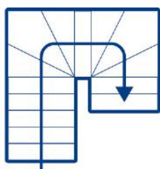
VTVT 2/4 tournant composé de trois volées et de deux quartiers
